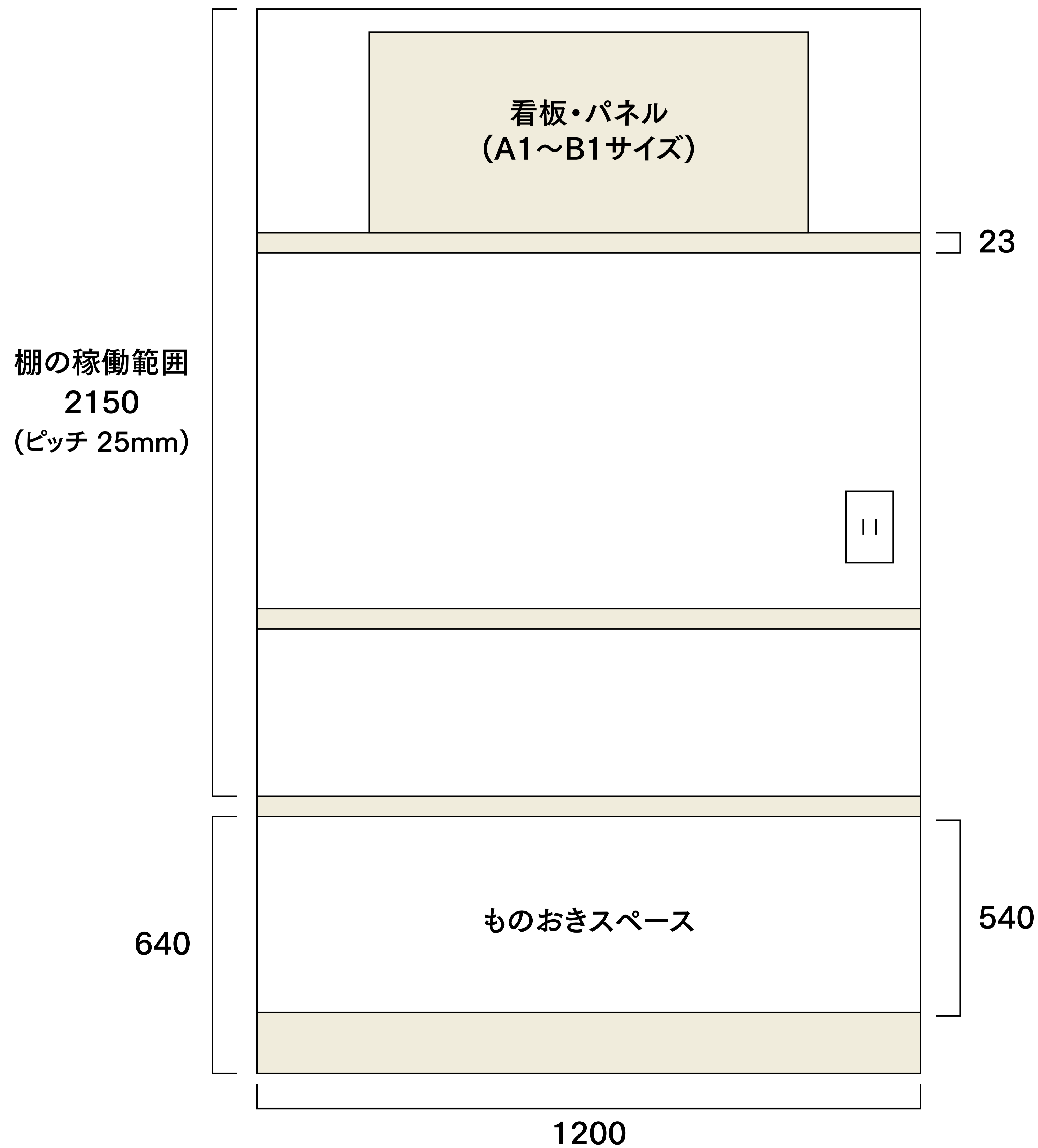
<正面図>
